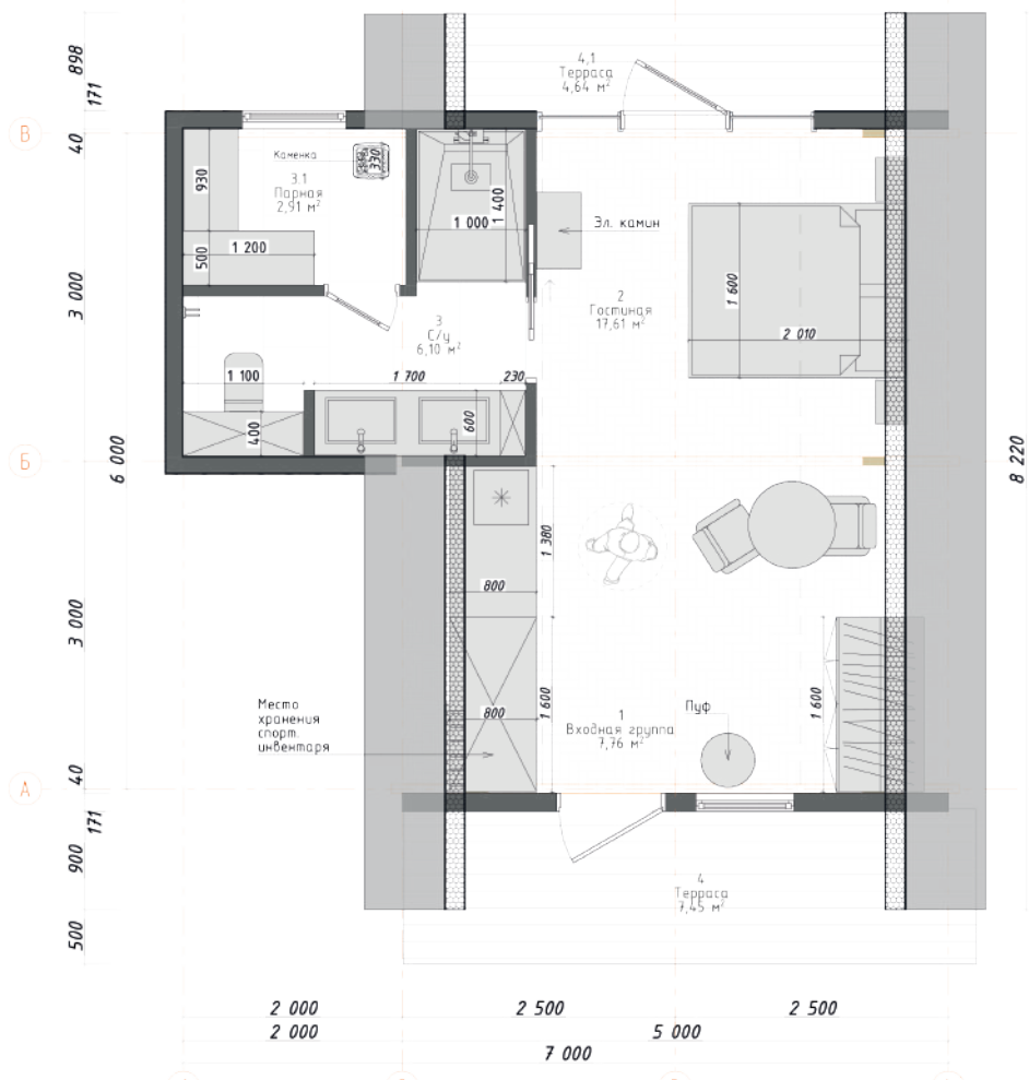
Планировочное решение
