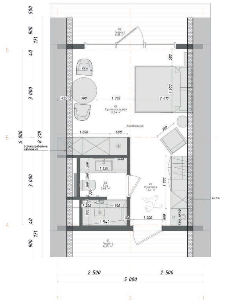
Планировочное решение
